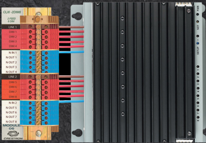
8路可控硅模块
